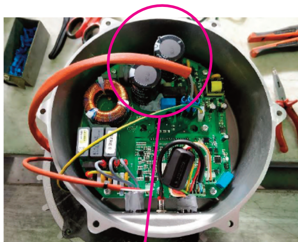
Condensadores electrolíticos
