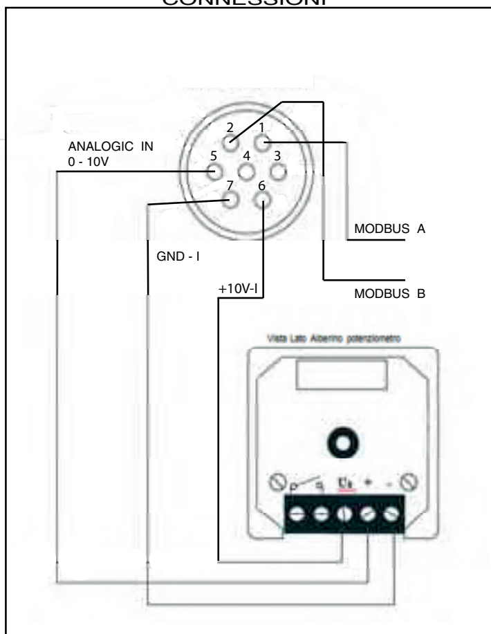
DETTAGLIO CONNESSIONI
