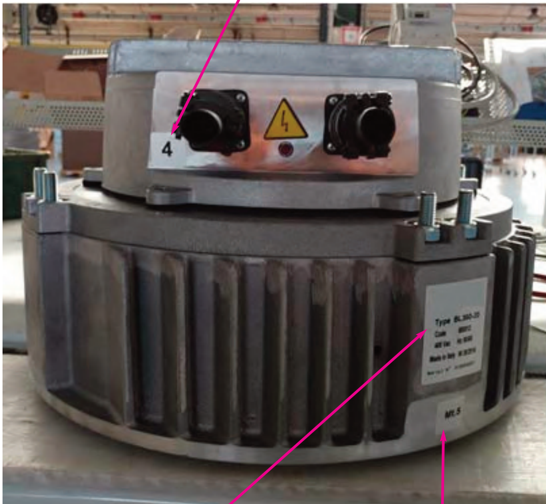
Etiqueta Modelo Moto-inversor y Número de Serie
