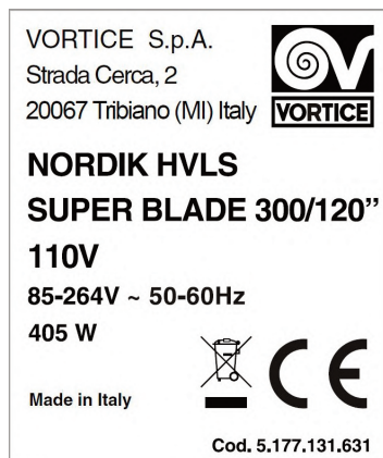
Fig. 1 - Ejemplo placa de datos para SUPERBLADE 300/120" 110V
